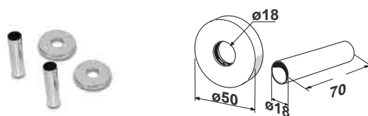
KIT COPRITUBO PER VALVOLE LUCIDE
