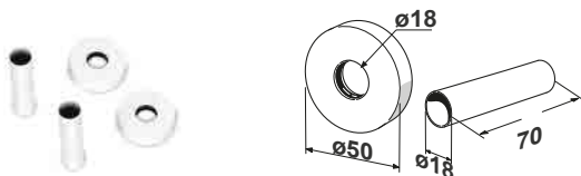
KIT COPRITUBO - SOLO UNITAMENTE ALLA VALVOLA ORDINABILE PER VALVOLE ELEGANT BIANCHE
