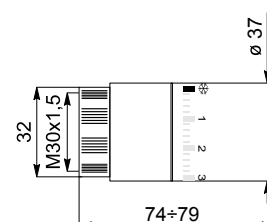
Testa termostatica a liquido BIANCA
