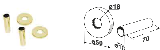
KIT COPRITUBO PER VALVOLE ORO ANTICO
