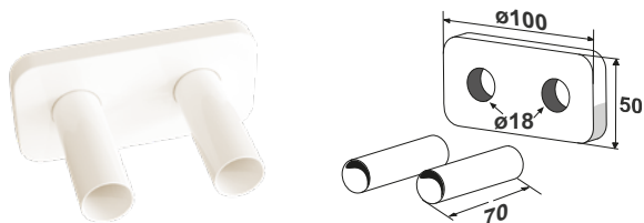
KIT COPRITUBO INT. 50 MM ORDINABILE PER VALVOLE ELEGANT BIANCHE
