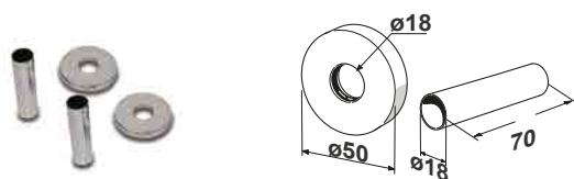
KIT COPRITUBO PER VALVOLE SATINATE
