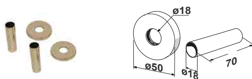
KIT COPRITUBO PER VALVOLE BRONZO ANTICO
