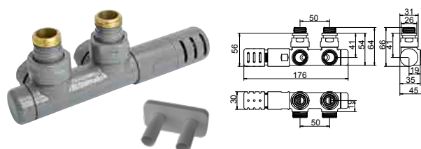
INTERASSE 50 MM A SQUADRA CON TESTA TERMOSTATICA DESTRA - per allacciamenti tipo V7 - V8 - V11
