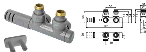
INTERASSE 50 MM A SQUADRA CON TESTA TERMOSTATICA SINISTRA - per allacciamenti tipo V7 - V8 - V11
