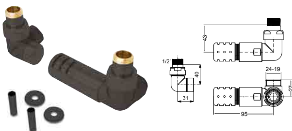
CORNER CON TESTA TERMOSTATICA DESTRA
