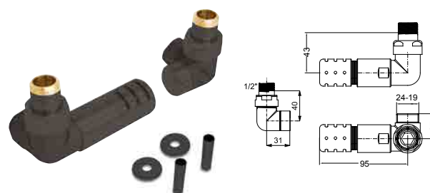
CORNER CON TESTA TERMOSTATICA SINISTRA
