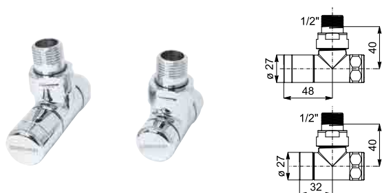
A SQUADRA MANUALE
