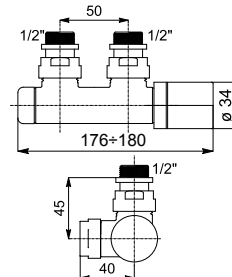
INTERASSE 50 MM A SQUADRA CON TESTA TERMOSTATICA DESTRA - per allacciamenti tipo V7 - V8 - V11
