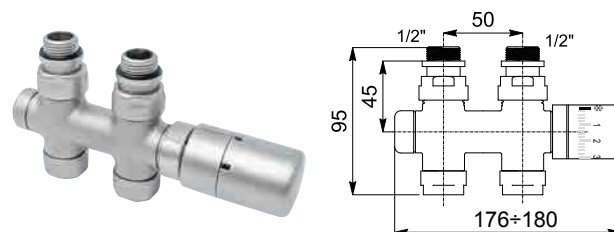
INTERASSE 50 MM DRITTA CON TESTA TERMOSTATICA per allacciamenti tipo V7 - V8 - V11
