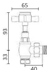
A SQUADRA MANUALE BRONZO ANTICO
