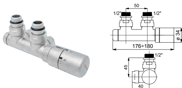
INTERASSE 50 MM A SQUADRA DESTRA per allacciamenti tipo V7 - V8 - V11
