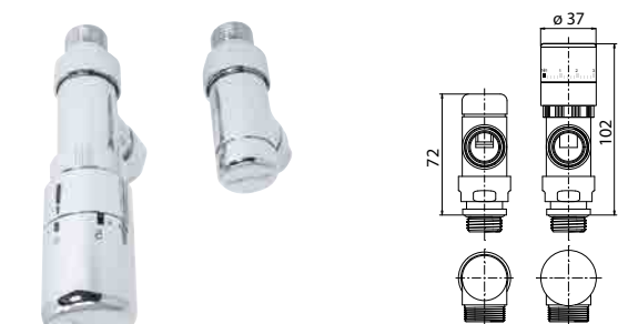
REVERSA CON TESTA TERMOSTATICA
