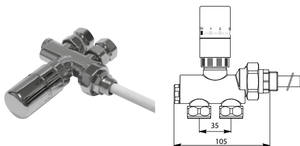
VANNE MONOTUBE AVEC TÊTE THERMOSTATIQUE CHORME pour raccordements de type V12 - V13
