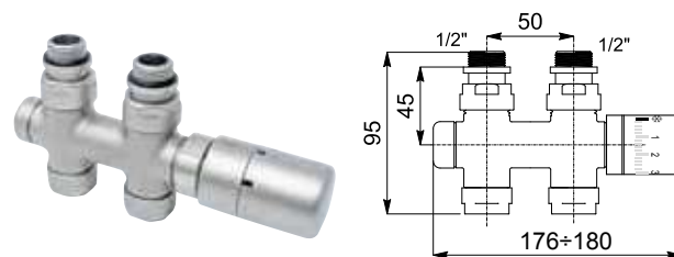
DURCHGANGSFORM INKL THERMOSTATKOPF N.A. 50 MM Für Anschlusstypen V7 - V8 - V11
