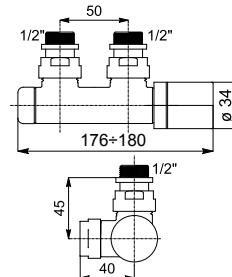
ECKFORM N.A. 50 MM INKL THERMOSTATKOPF (RECHTS)
