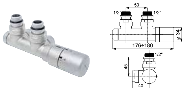
ECKFORM N.A. 50 MM INKL THERMOSTATKOPF (RECHTS) Für Anschlusstypen V7 - V8 - V11
