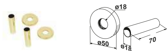
ROHRABDECKUNGSSETS
