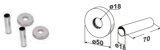
ROHRABDECKUNGSSETS
