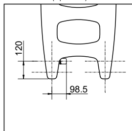
Thermostatkopf-Positionierung (optional)
