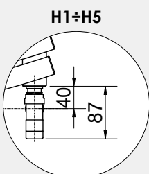
Abmessungen Ventilset Cordivari Elegant Reverse manuell
