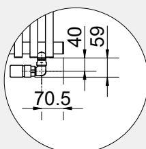
Abmessungen Ventilset Cordivari Elegant Corner mit Therstatkopf
